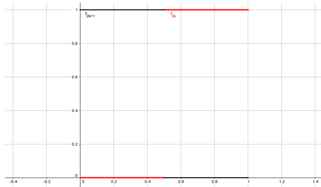
Figura 1.6: f_n(x)
