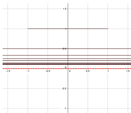
Figura 1.7: f_n(x)
