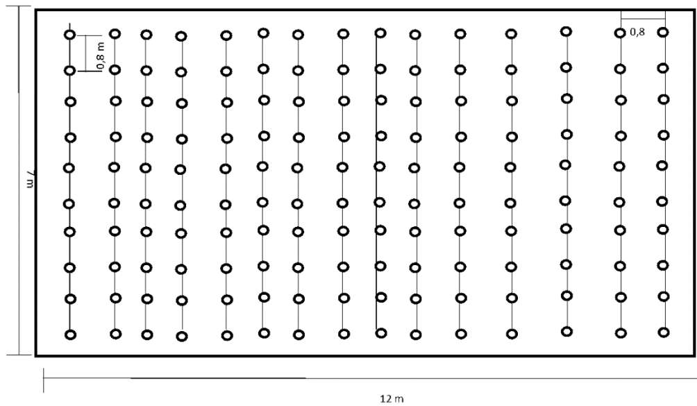
Figura 5: Diseño de la distribución en planta en línea de la huerta urbana en Sierra Morena, Bogotá
