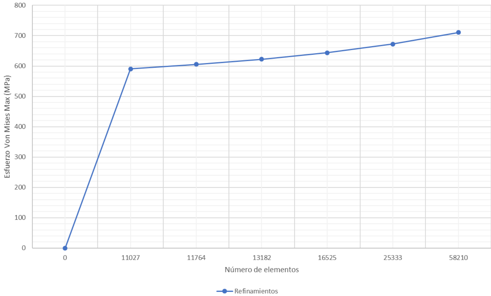
Número de elementos vs Esfuerzo Von mises
