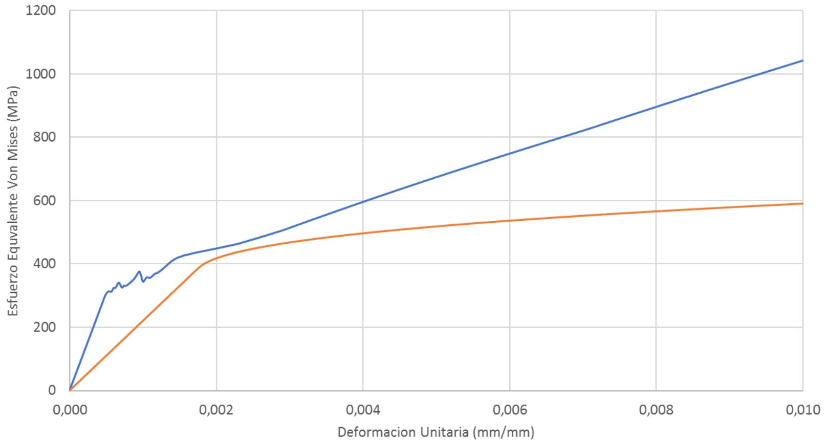
Promedio Probeta 02 Esfuerzo Vs Deformación
