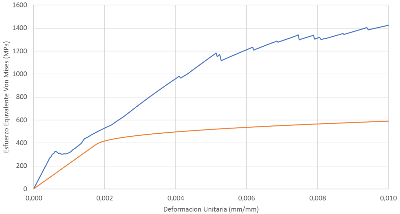
Promedio Probeta 04 Esfuerzo Vs Deformación
