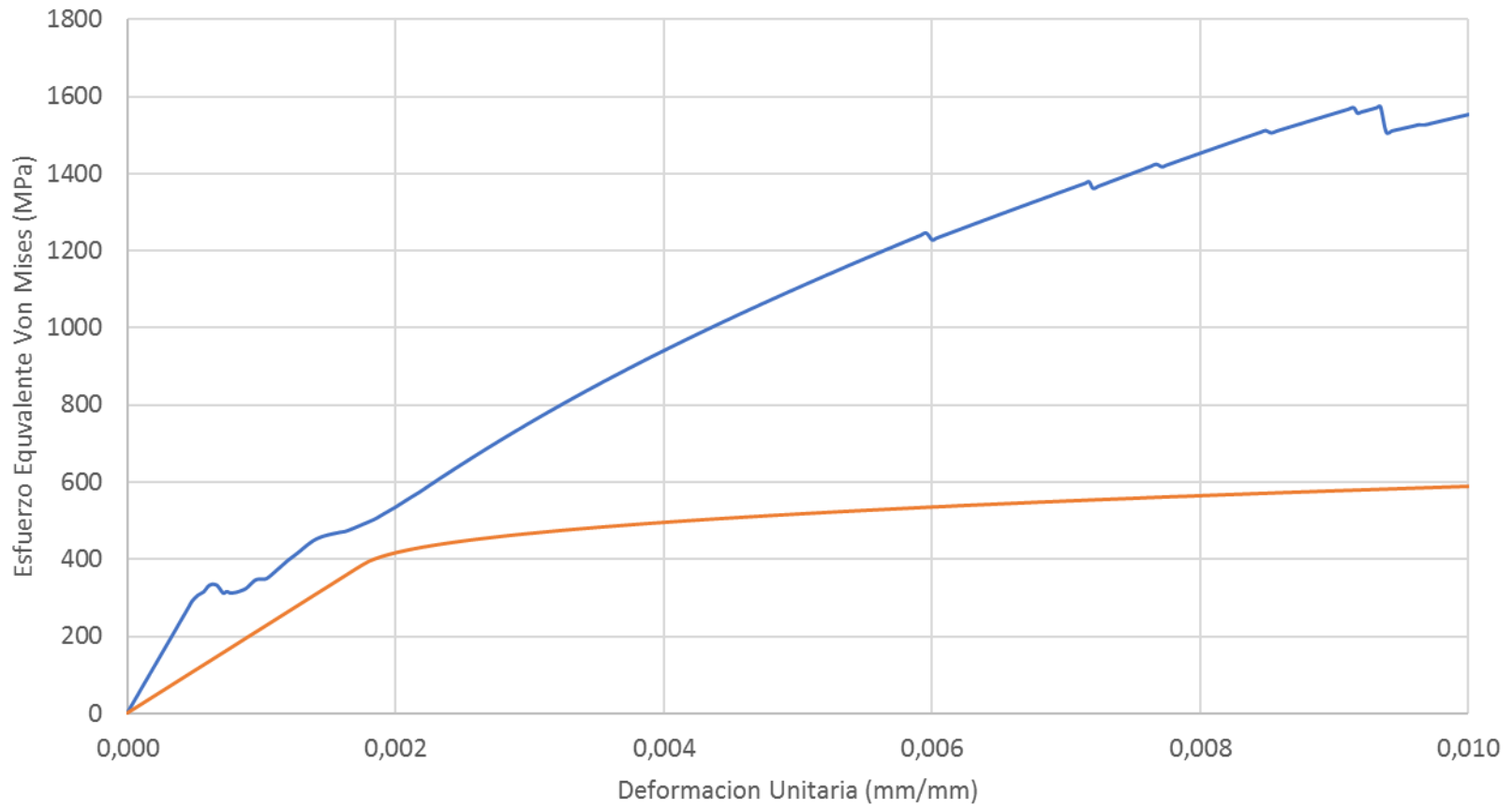
Promedio Probeta 08 Esfuerzo Vs Deformación
