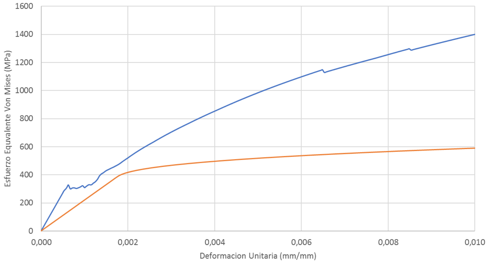
Promedio Probeta 06 Esfuerzo Vs Deformación
