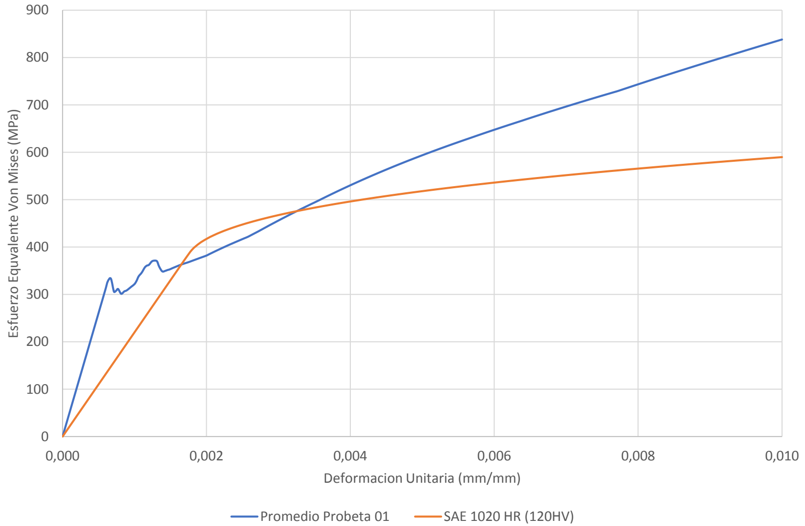
Promedio Probeta 01 Esfuerzo Vs Deformación
