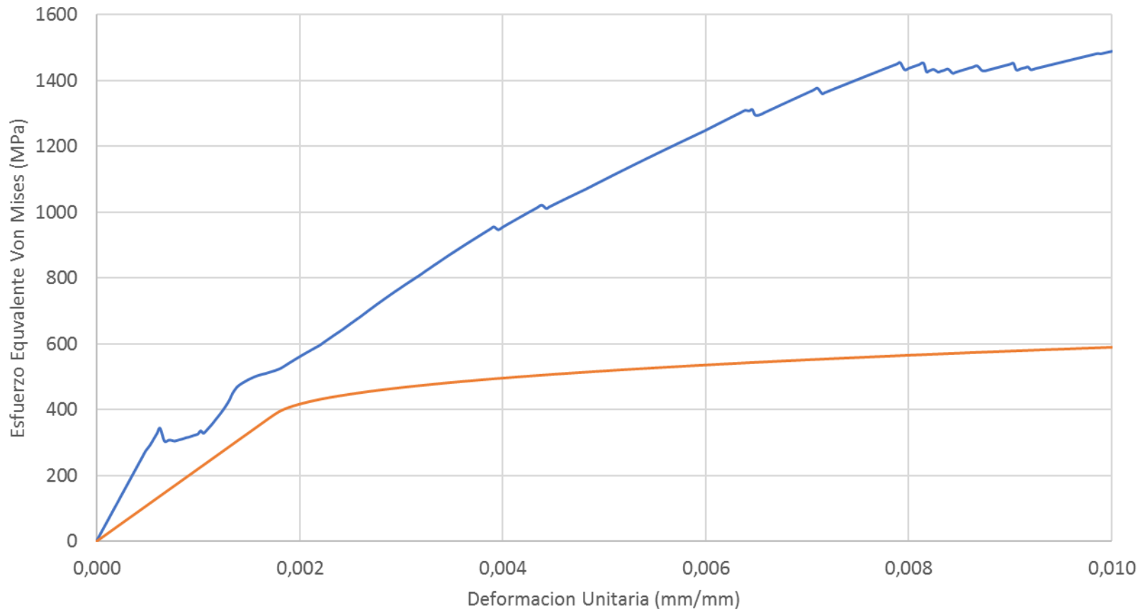
Promedio Probeta 07 Esfuerzo Vs Deformación
