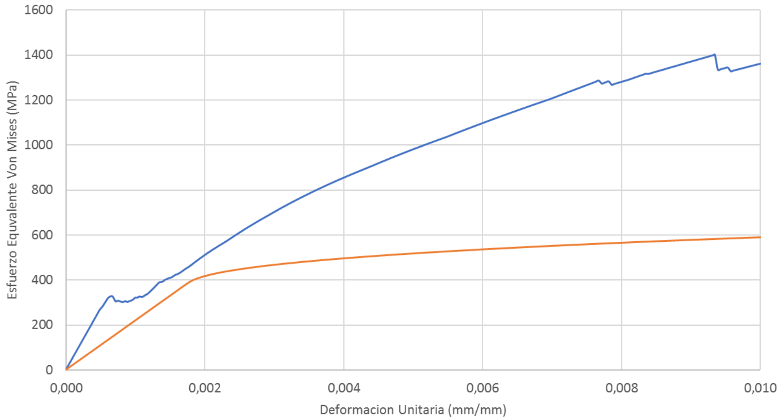
Promedio Probeta 05 Esfuerzo Vs Deformación
