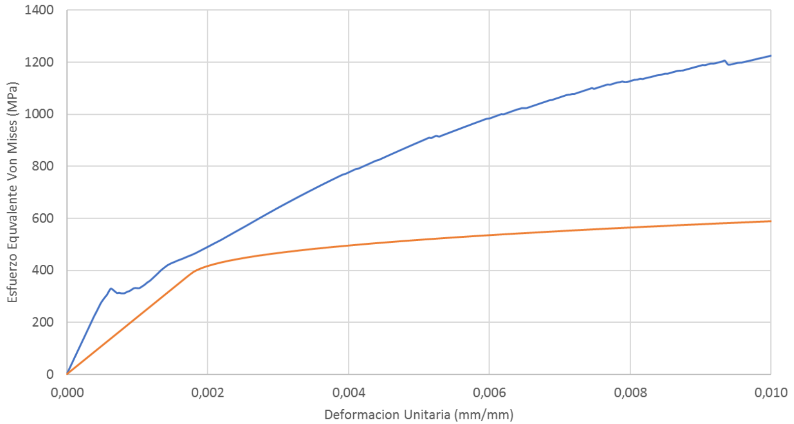
Consolidado SAE 1020 + TT Esfuerzo Vs Deformación
