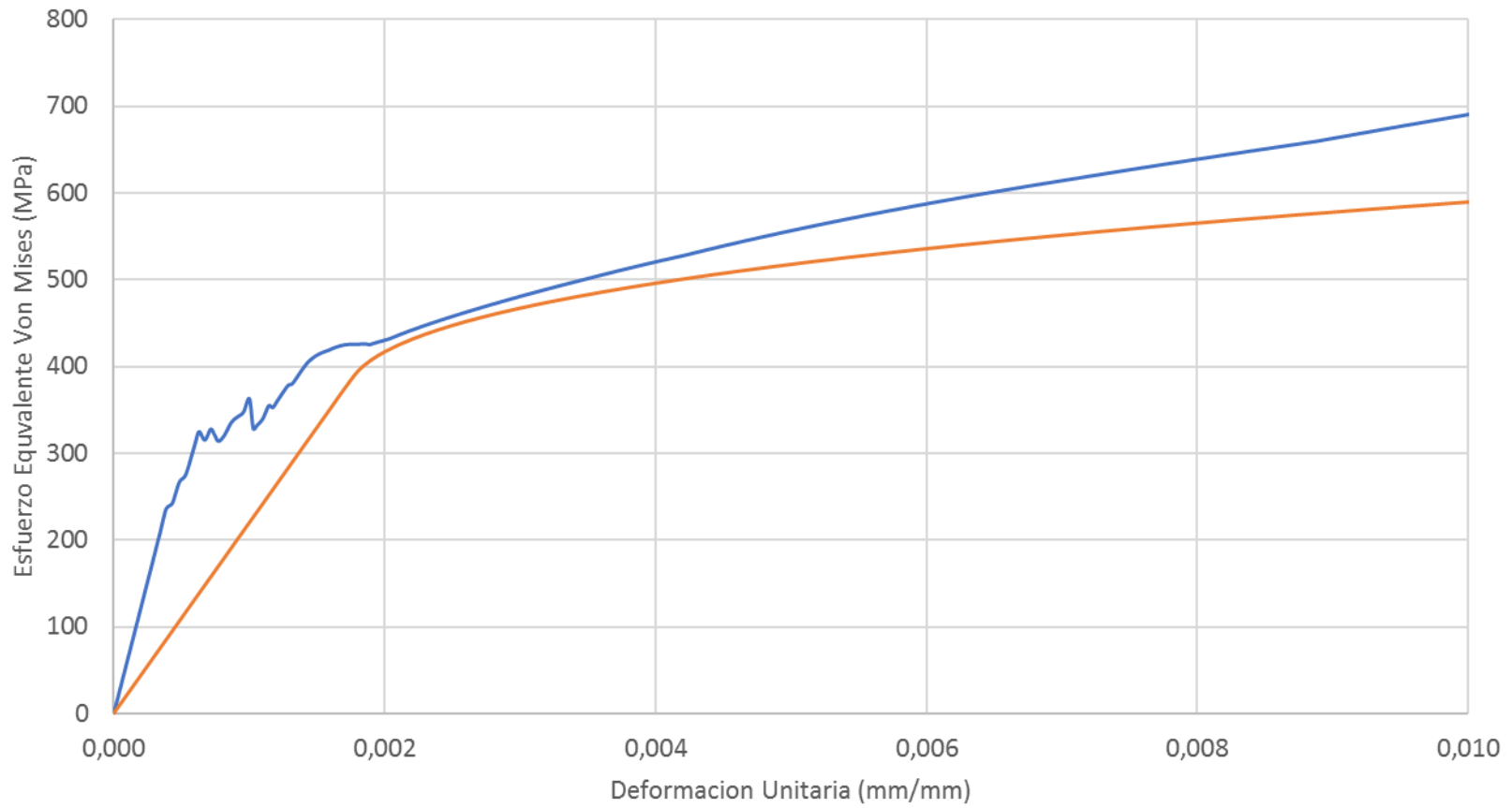
Promedio Probeta 03 Esfuerzo Vs Deformación
