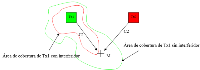
Figura 2 Víctima, interferidor y receptor
